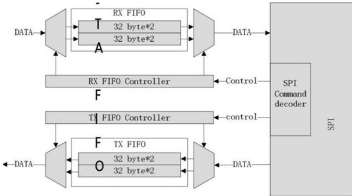
FIFO 框图
